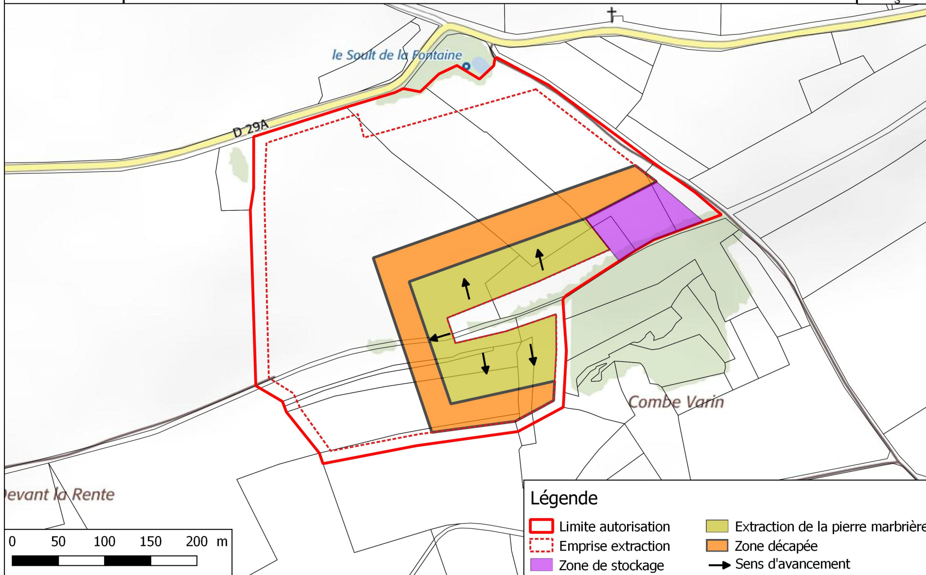
Figure 9 : Phasage d'extraction - Phase 1
