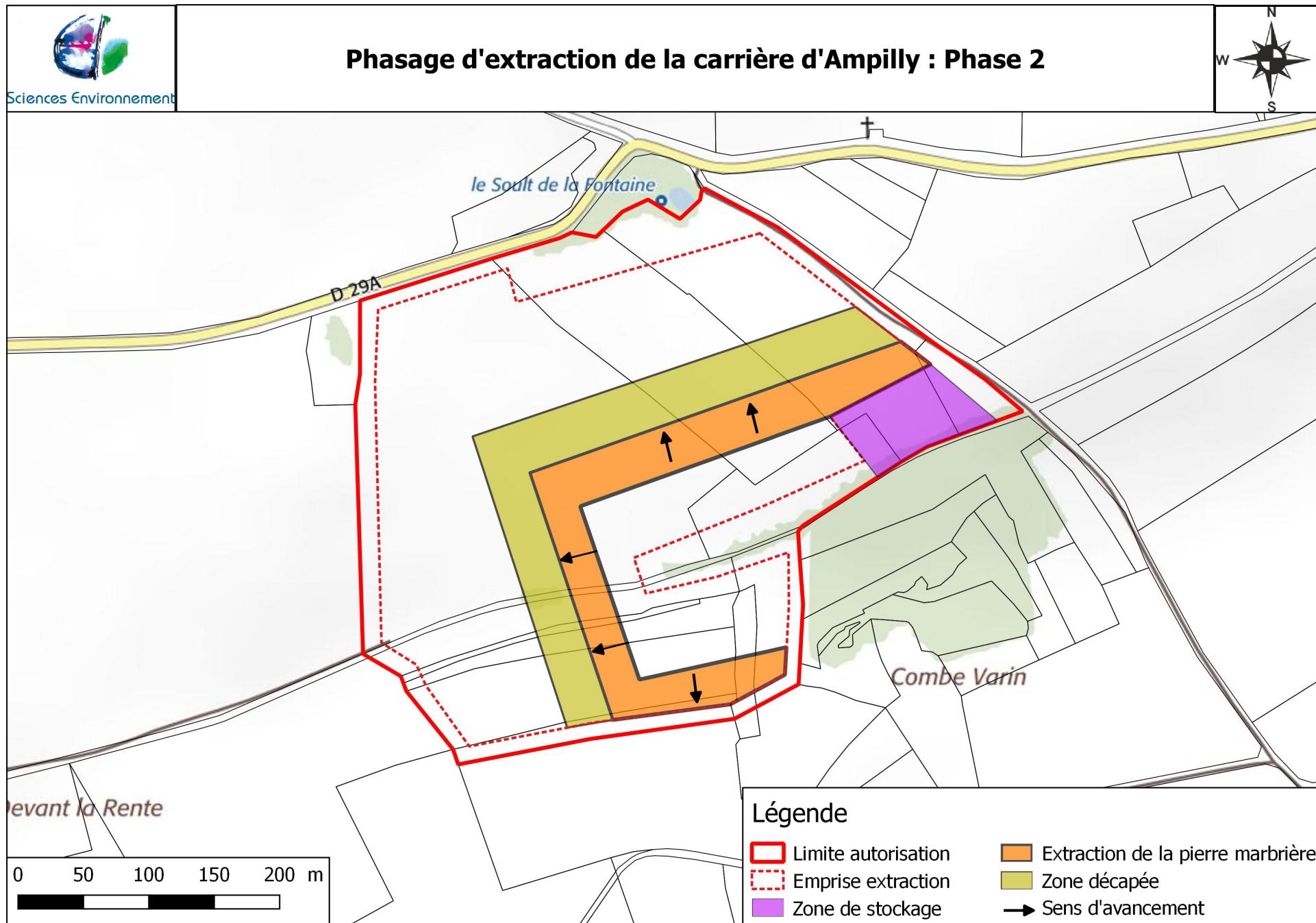
Figure 10 : Phasage d'extraction - Phase 2
