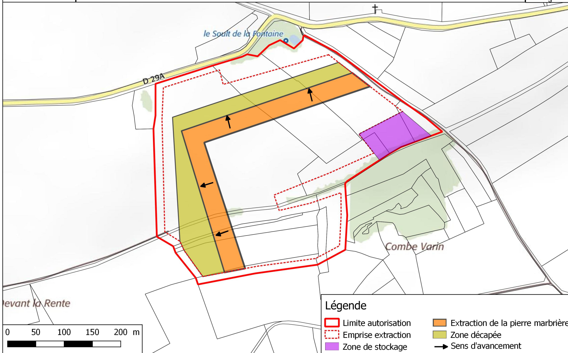
Figure 12 : Phasage d'extraction - Phase 4
