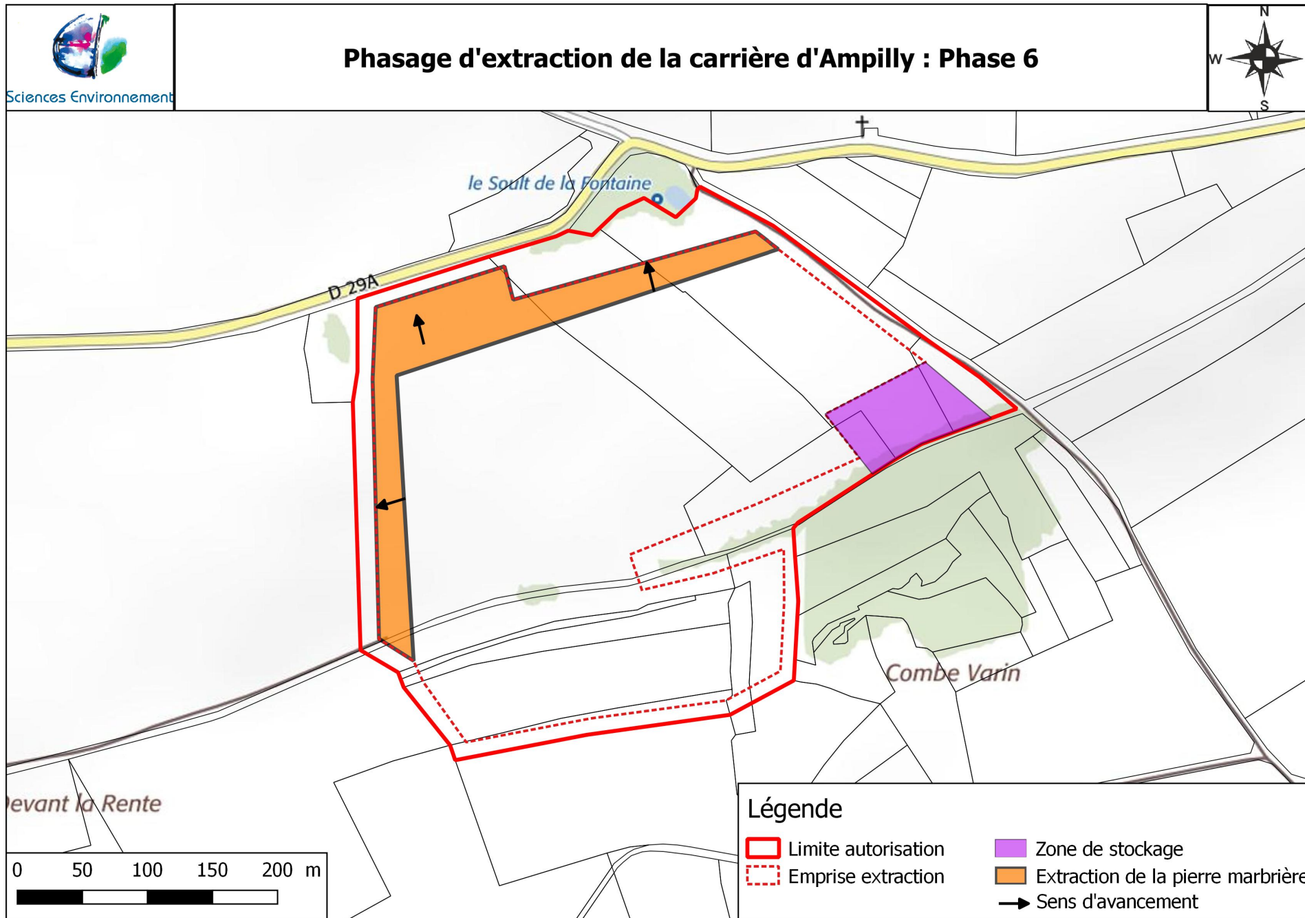
Figure 14 : Phasage d'extraction - Phase 6
