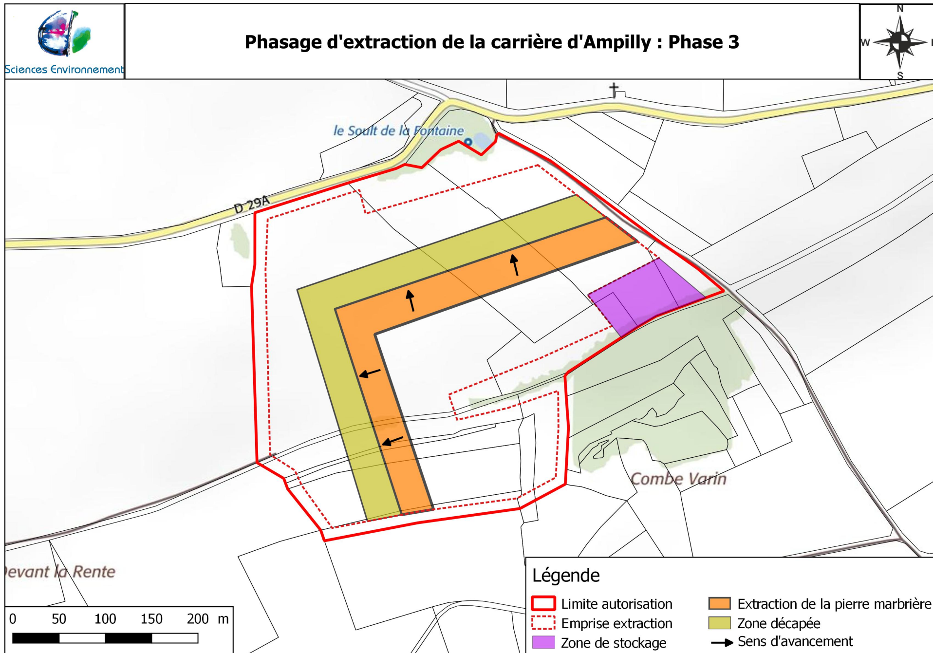
Figure 11 : Phasage d'extraction - Phase 3
